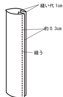
図B ピンタックの縫い方
